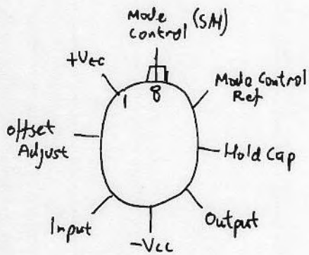
SHC298 Sample/Hold
